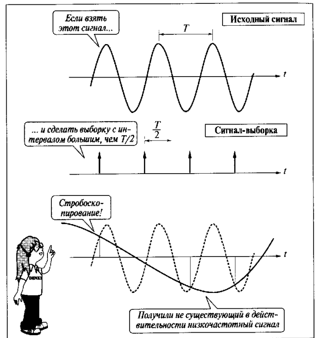
Рис. 1.10. Что такое стробоскопирование
