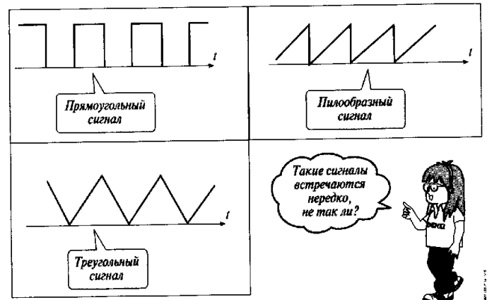
Рис. 1.4. Основные виды периодических сигналов
