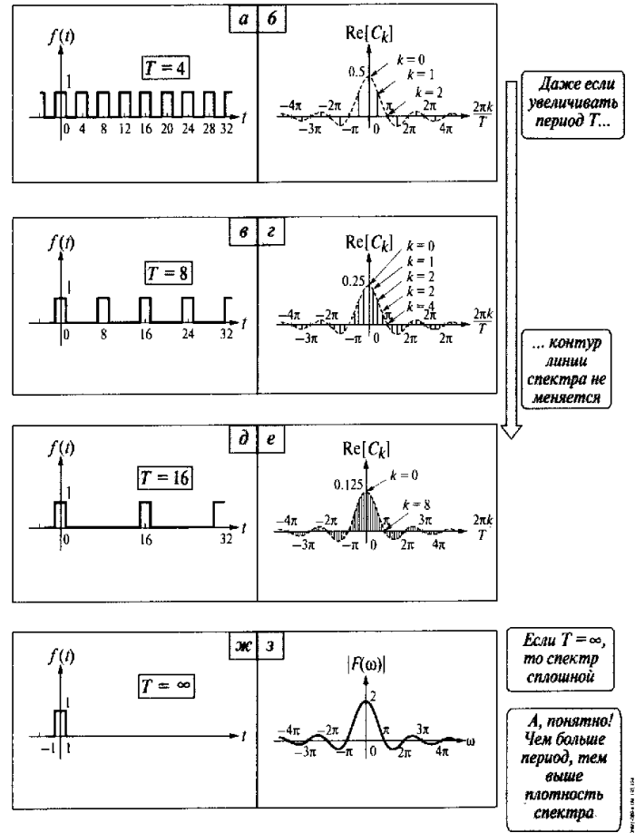
Рис. 7.2. Спектр последовательности прямоугольных импульсов
