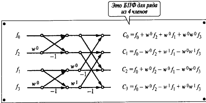
Рис. 6.8. БПФ для ряда из 4 членов
