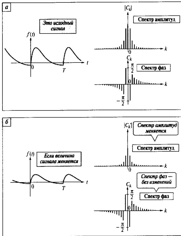
Рис. 5.20. Связь между величиной сигнала и спектра
