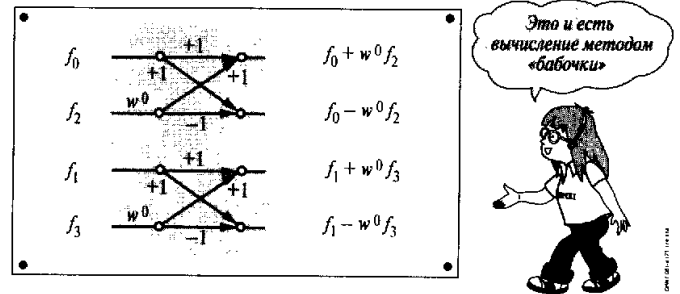
Рис. 6.7. Метод вычисления «бабочкой»
