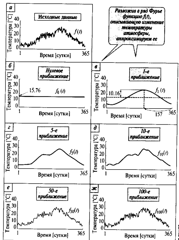
5.16. Аппроксимация функции с помощью ряда Фурье
