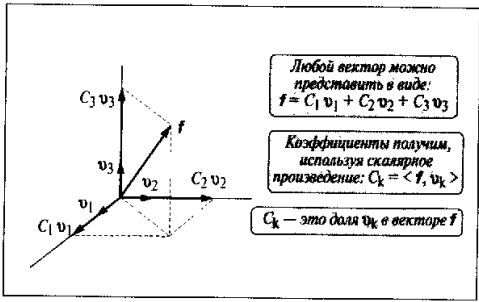
Рис. 3.9. Выражение вектора 3-мерного пространства через ортонормированный базис
