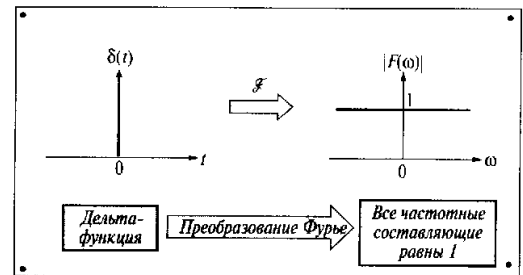
Рис. 7.7. Спектр дельта-функции
