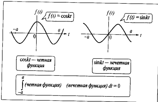
Рис. 5.5. Интегрирование произведения четной и нечетной функций
