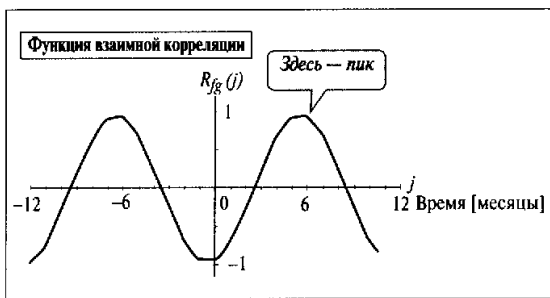
Рис. 4.4. Функция взаимной корреляция температуры Токио и Буэнос-Айреса
