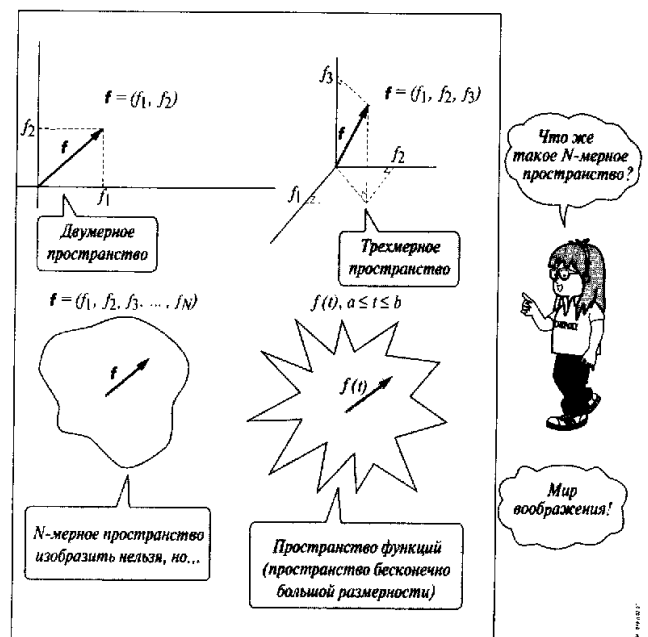
Рис. 3.2. Векторное пространство и пространство функций
