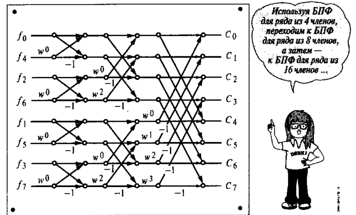
Рис. 6.10. Схема алгоритма БПФ для ряда из 8 членов
