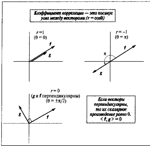
Рис. 3.6. Коэффициент корреляции
