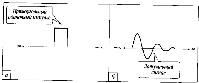
Рис. 1.5. Виды сигналов
