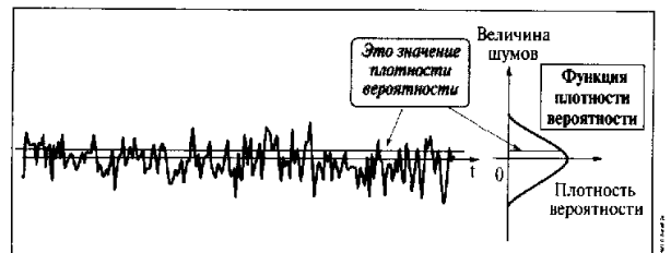
Рис. 2.5. Гауссовское свойство шумов
