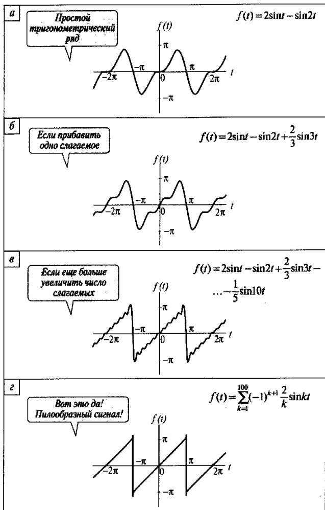
Рис. 5.1. Суммирование членов некоторого тригонометрического ряда
