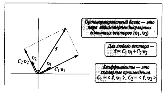
Рис. 3.7. Выражение вектора через ортонормированный базис
