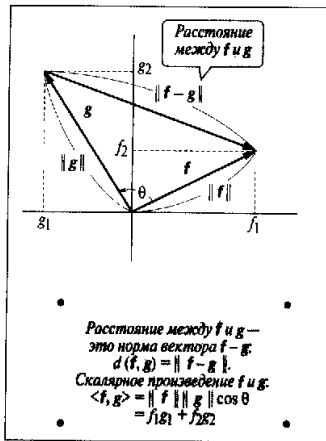
Рис. 3.4. Расстояние и скалярное произведение двумерных векторов
