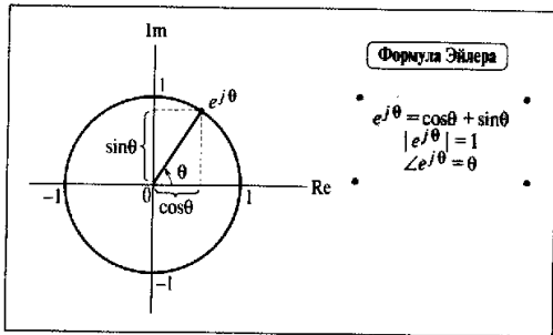
Рис. 5.8. Графическая иллюстрация формулы Эйлера
