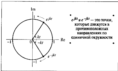
Рис. 5.12. Что такое e^{jkt} и e^{-jkt}
