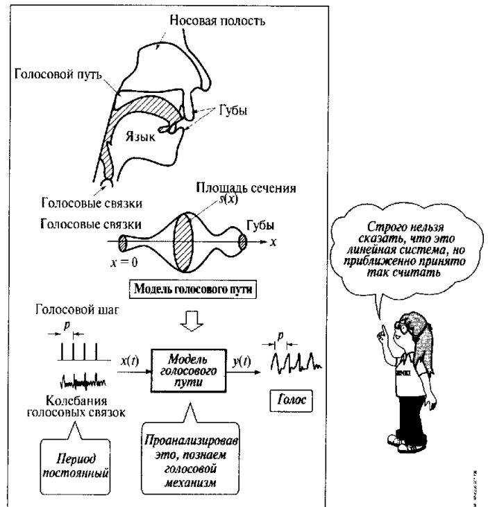
Рис. 8.3. Модель возникновения голосового звука
