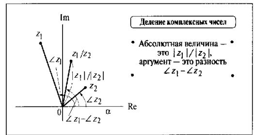
Рис. 5.11. Деление двух комплексных чисел
