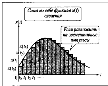
Рис. 8.4. Попробуем разбить сигнал на элементарные импульсы
