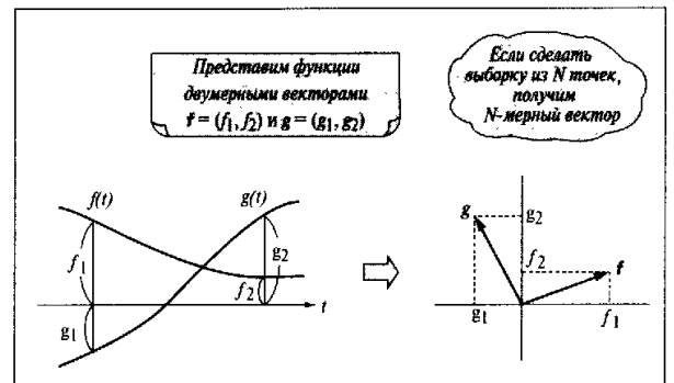
Рис. 3.3. Векторное выражение функции
