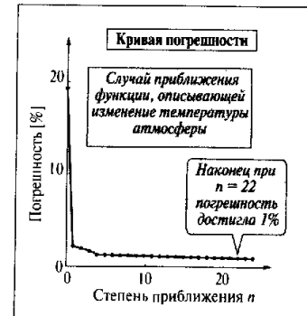
Рис. 5.17. Погрешность приближения для сложного сигнала
