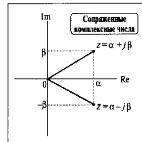
Рис. 5.7. Представление сопряженных комплексных чисел
