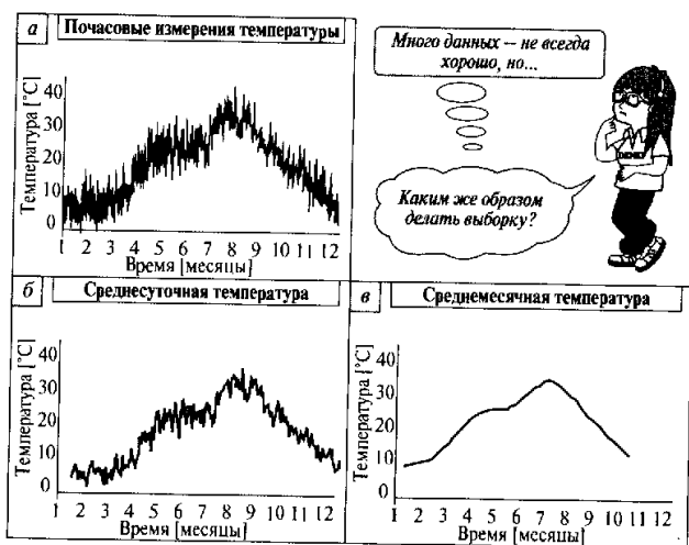
Рис. 1.7. Выборка изменений температуры атмосферы
