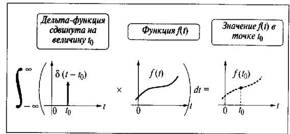
Рис. 7.6. Выражение выборки математической формулой
