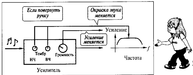
Рис. 8.2. Попробуем исследовать линейную систему
