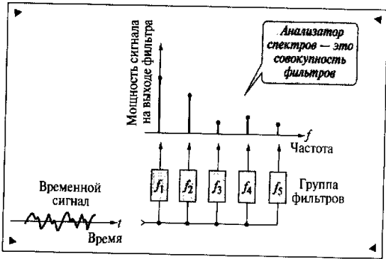
Рис. 6.1. Анализатор спектра
