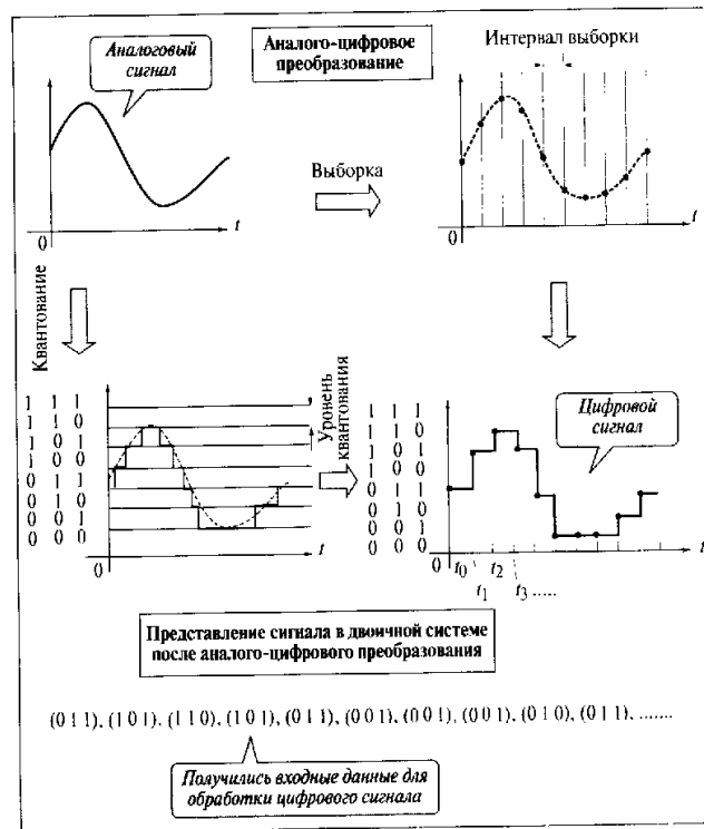
Рис. 1.6. Преобразование аналогового сигнала в цифровой
