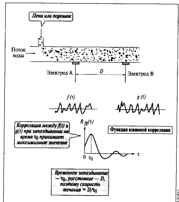
Рис. 4.5. Измерение скорости течения с помощью функции взаимной корреляции
