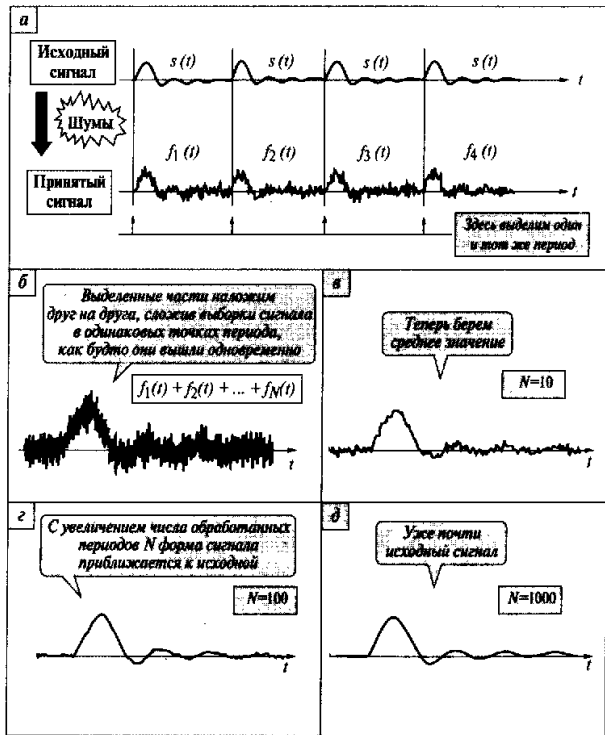
Рис. 2.4. Подавление шумов
