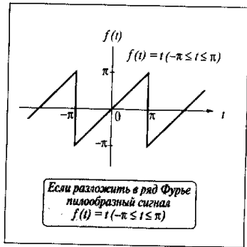
Рис. 5.3. Сигнал пилообразной формы
