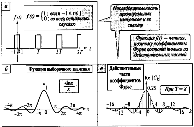
Рис. 5.14. Последовательность прямоугольных импульсов и ее спектр
