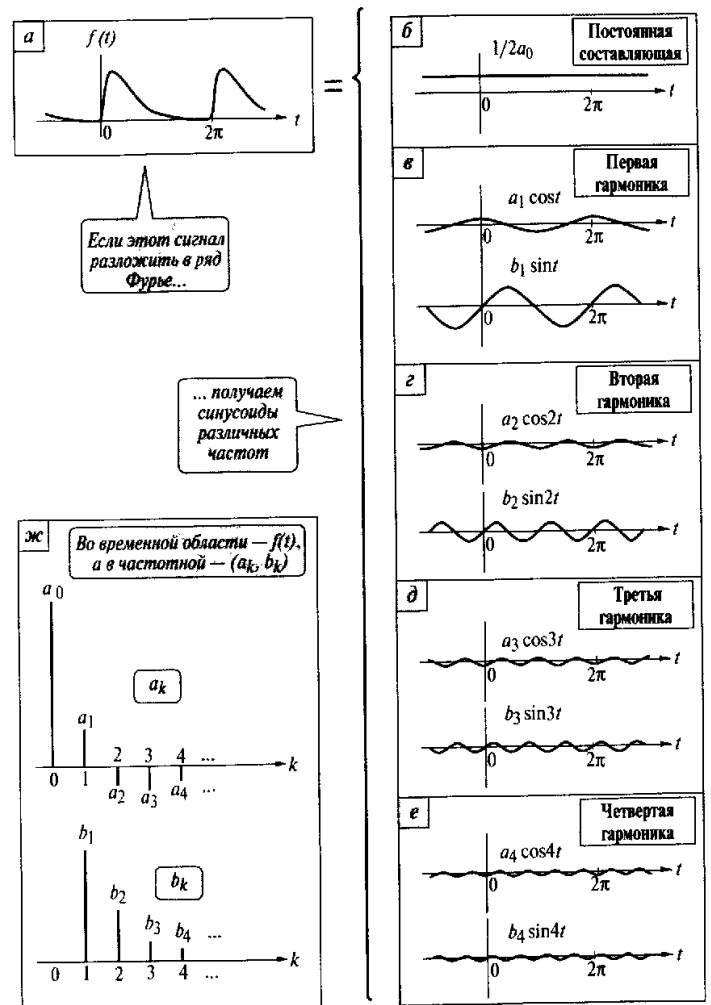
Рис. 5.2. Разложение сигнала
