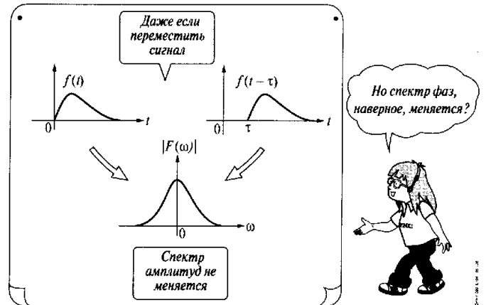
Рис. 7.3. Что происходит при сдвиге сигнала во времени
