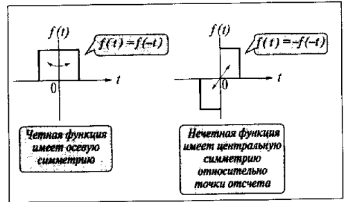
Рис. 5.4. Четные и нечетные функции
