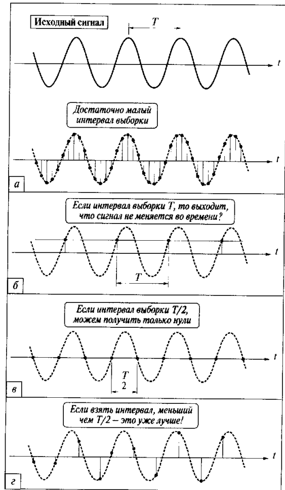
Рис. 1.9. Выборка синусоиды
