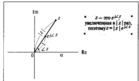
Рис. 5.9. Выражение произвольного комплексного числа через модуль и аргумент
