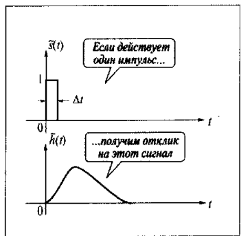
Рис. 8.5. Рассмотрим только один импульс
