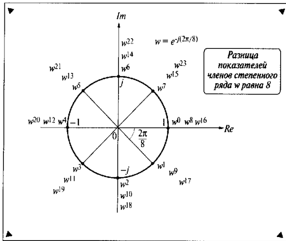
Рис. 6.5. Степенной ряд w
