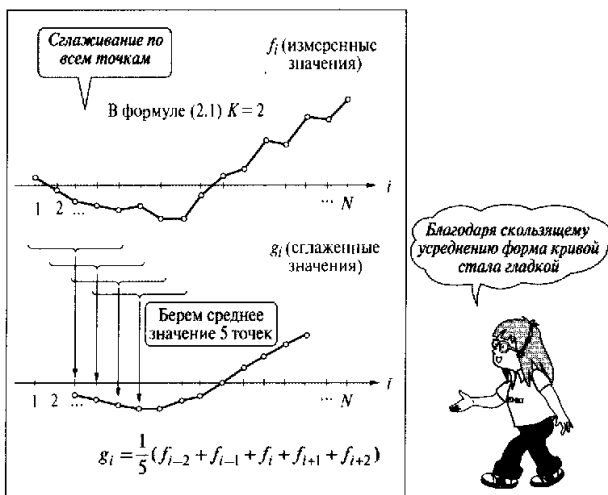
Рис. 2.1. Методика нахождения скользящего среднего
