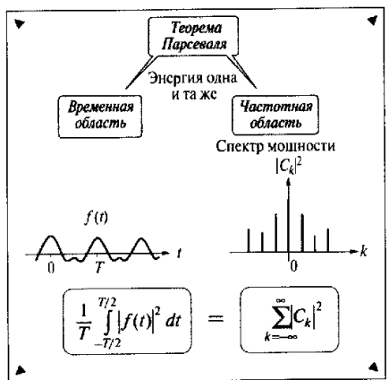
Рис. 5.15. Теорема Парсевала
