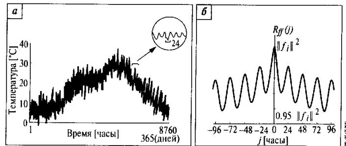
Рис. 4.7. Функция автокорреляции температуры атмосферы
