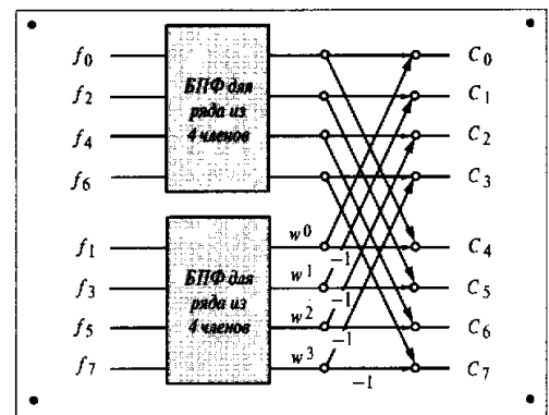
Рис. 6.9. БПФ для ряда из 8 членов с использованием БПФ для ряда из 4 членов
