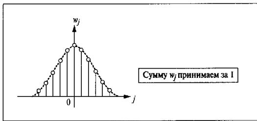
Рис. 2.3. Пример весовой функции (распределение Гаусса)
