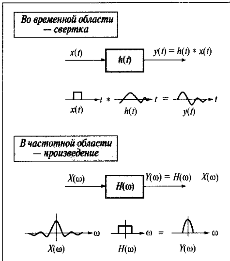
Рис. 8.9. Как описывается линейная система
