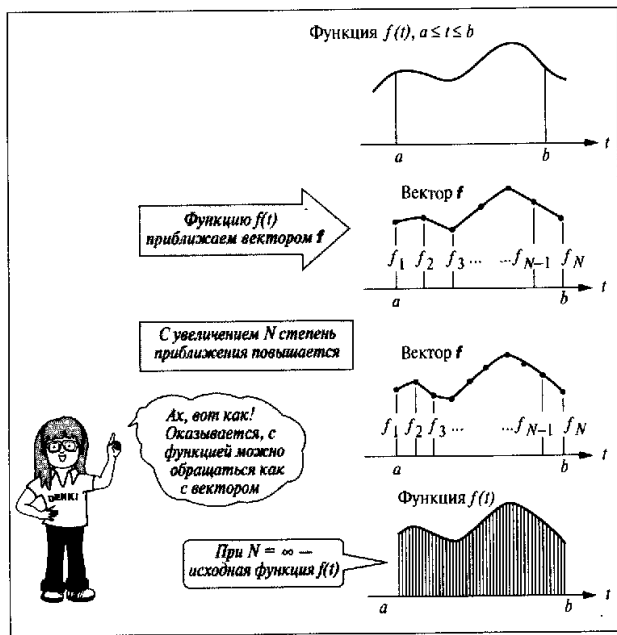
Рис. 3.1. Векторное представление функции
