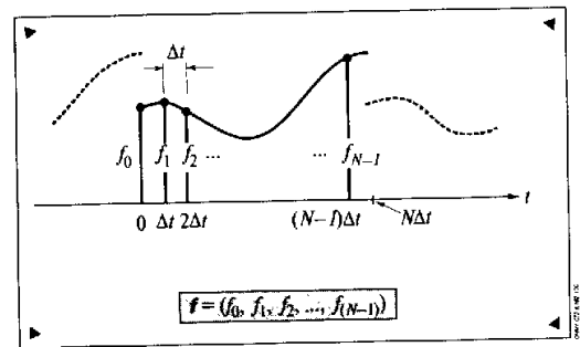
Рис. 6.2. N значений сигнала
