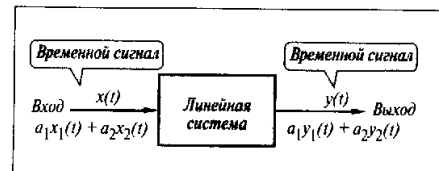
Рис. 8.1. Попробуем исследовать линейную систему
