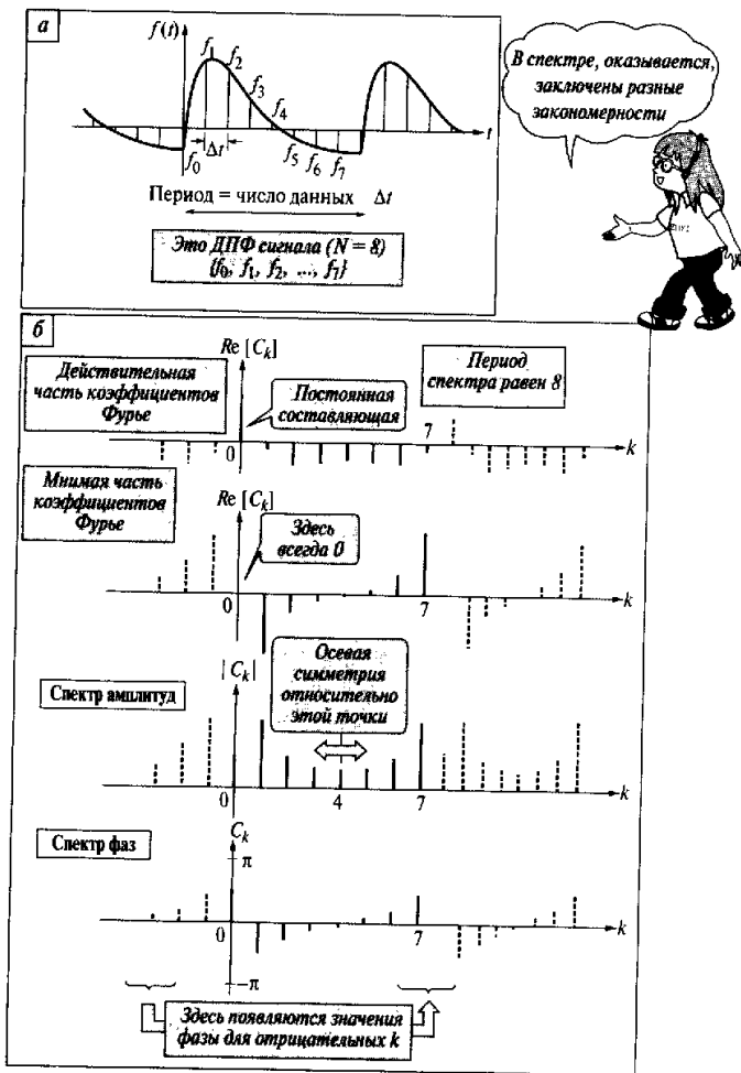
Рис. 6.4. Спектры ДПФ
