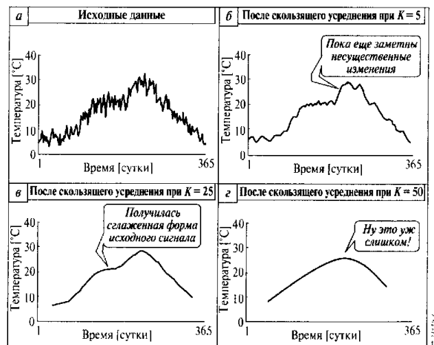
Рис. 2.2. Сглаживание графиков температуры атмосферы методом скользящего среднего
