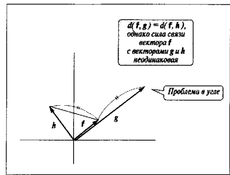
Рис. 3.5. Связь между векторами
