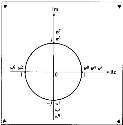
Рис. 6.6. Степенной ряд w для N = 4
