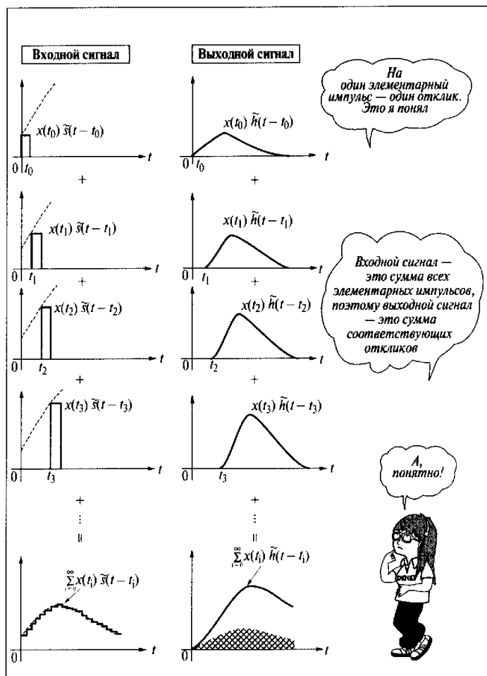
Рис. 8.6. Суммарный входной сигнал и суммарный выходной сигнал
