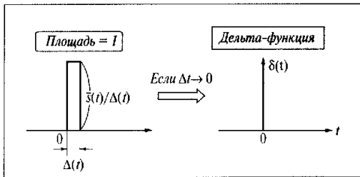
Рис. 8.7. Что такое дельта-функция
