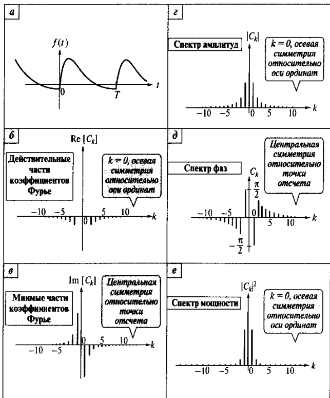
Рис. 5.13. Спектры и комплексные коэффициенты Фурье
