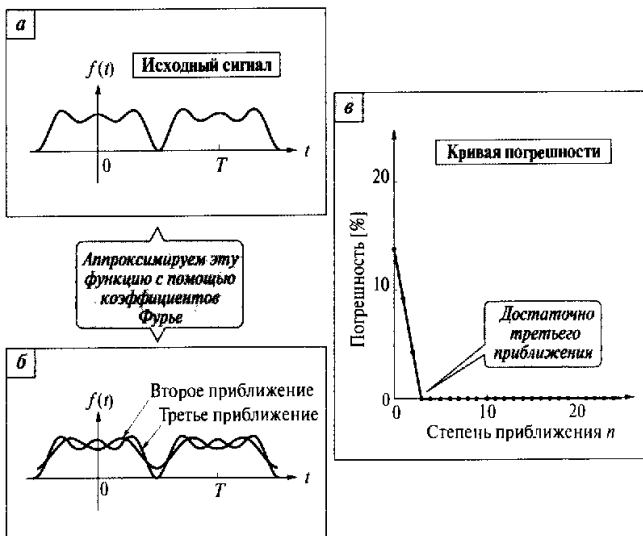
Рис. 5.18. Разложение в ряд Фурье гладкой функции
