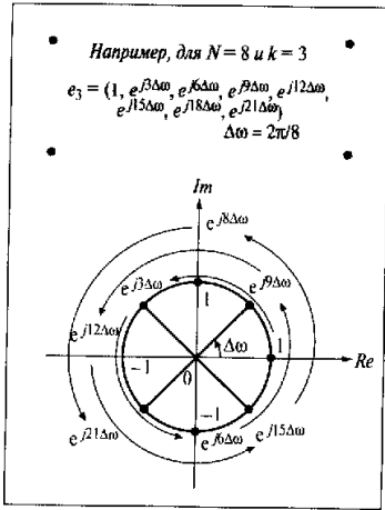
Рис. 6.3. Базисный N -мерный вектор
