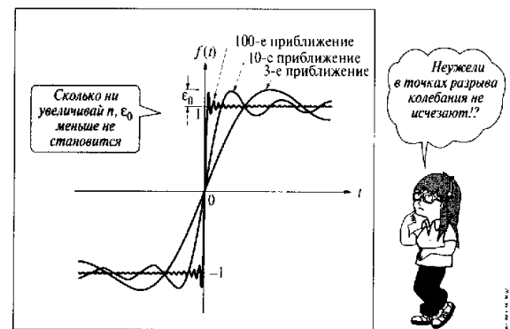
Рис. 5.19. Явление Гиббса
