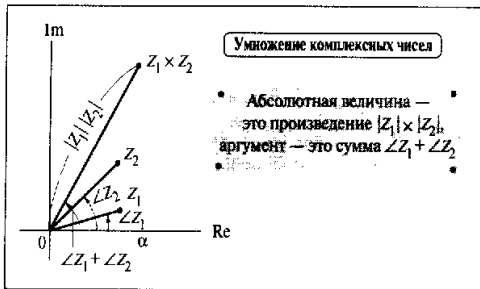
Рис. 5.10. Умножение двух комплексных чисел
