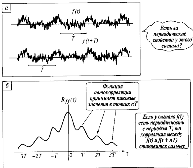
Рис. 4.6. Функция автокорреляции
