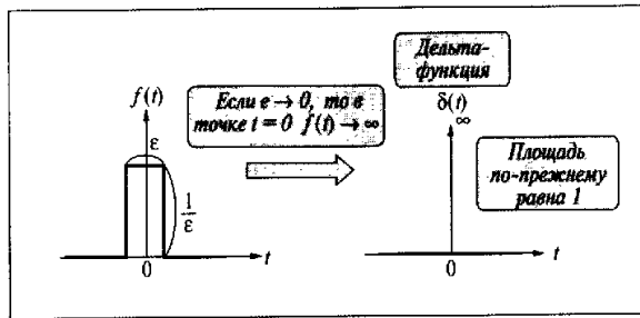
Рис. 7.5. Дельта-функция
