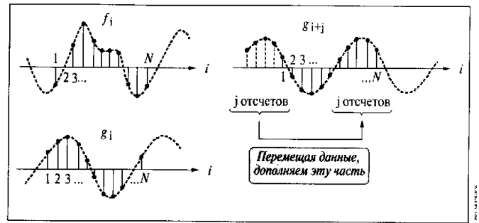
Рис. 4.3. Дополнение данных
