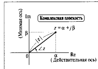
Рис. 5.6. Комплексное представление чисел на плоскости
